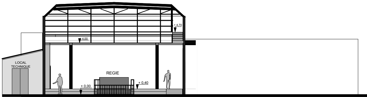
COUPE TRANSVERSALE
